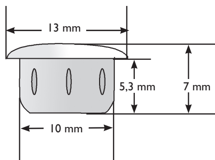
Réf.: I013 pour trou de 10 mm
