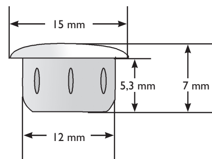
Réf.: I215 pour trou de 12 mm
